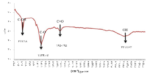
شکل 2- الف طیف FT-IR گلیکوزآمینوگلیکان‌های استخراج شده خام غضروف کوسه
