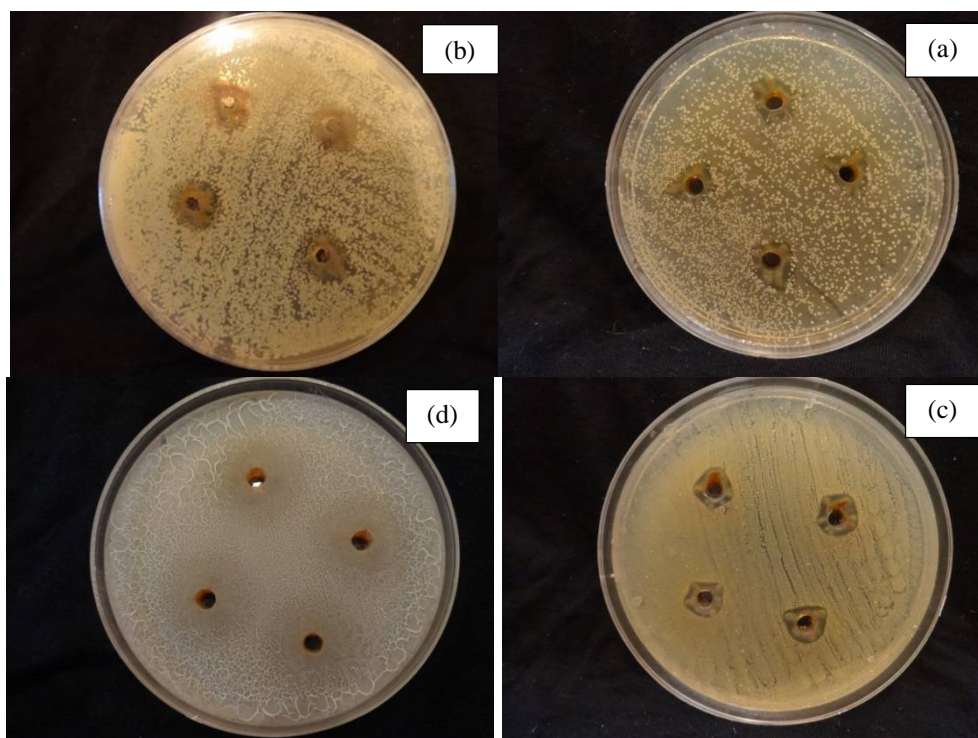
شکل 6 هاله عدم رشد به روش چاهک، (a) B. subtilis (b) S. cerevisiae (c) E. coli (d) S. aureus
