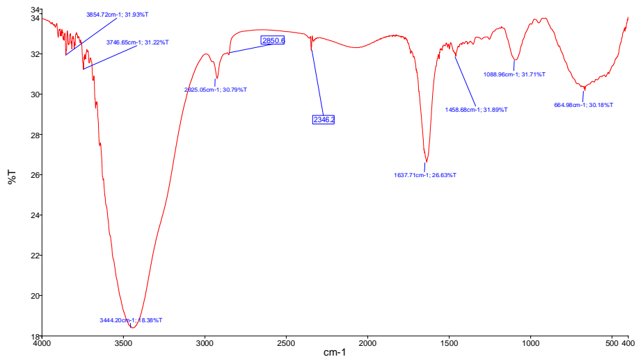
شکل 8- طیف FTIR سامانه لیپوزومی حاوی عصاره خار مریم
