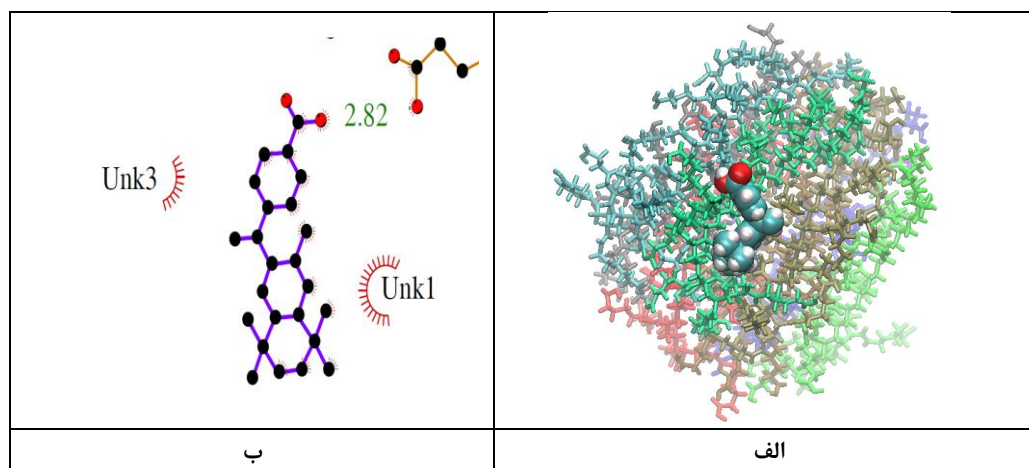
شکل ۳ الف) موقعیت لیگاند و هیدروژل نسبت به یکدیگر و ب) پیوند هیدروژنی مابین داروی بی کالوتامید و زنجیر شماره یک هیدروژل. داروی مورد مطالعه دارای گروه های عاملی متعدد می باشد که توانایی برقراری پیوند هیدروژنی را دارند. برقراری پیوندهای هیدروژنی درون و بین مولکولی در داخل ساختار هیدروژل موجب شده است تا فقط یک پیوند هیدروژنی مابین دارو و هیدروژل تشکیل شود.
