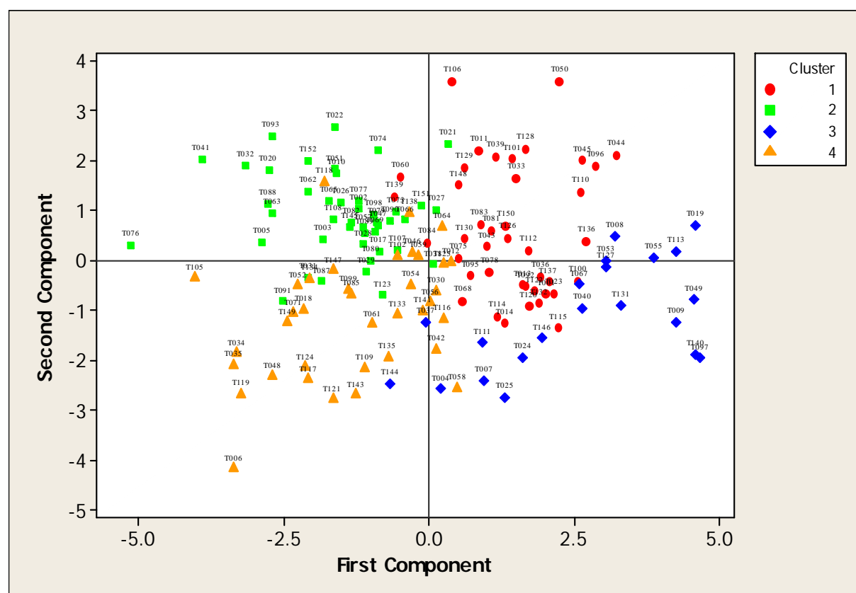
شکل 5 دسته‌بندی لاین‌های آفتابگردان روغنی بر اساس دو مؤلفه اول و دوم تجزیه به مؤلفه‌های اصلی روی صفات زراعی و مورفولوژیک
