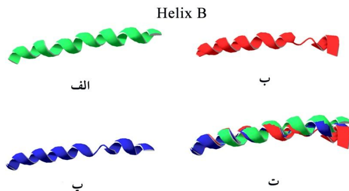
شكل 6 الف: ساختار مارپيچ B در لحظه اول، ب: ساختار مارپيچ B در لحظه مياني، پ: ساختار مارپيچ B در لحظه پاياني، ت: همرديفي ساختاري مارپيچ B در لحظات اول، مياني و پاياني
