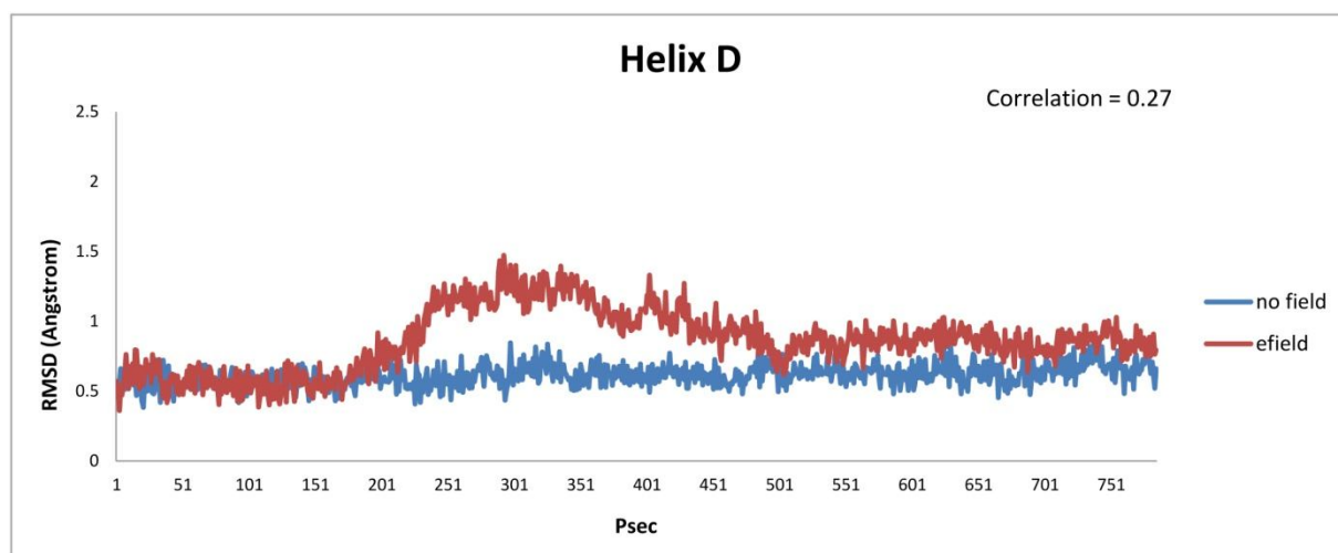
شکل 11 انحراف جذر میانگین مربعات کربن آلفا پس از اعمال میدان بر مارپیچ D در ساختار پروتئین تریمر درون غشای لیپیدی به مدت 786 پیکوثانیه معادل یک تناوب سینوسی
