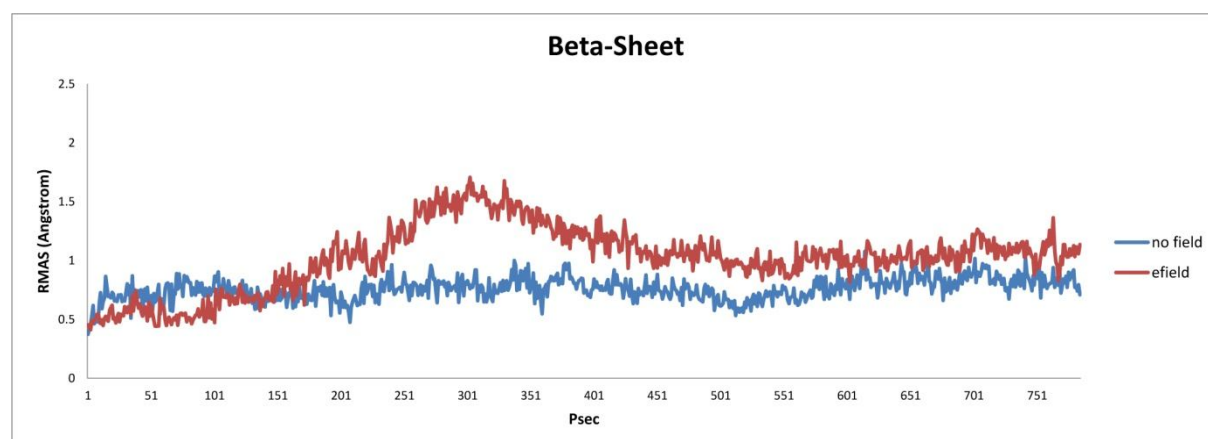
شكل 7 انحراف جذر ميانگين مربعات كربن آلفا پس از اعمال ميدان براي صفحه بتا در ساختار پروتئين تريمر درون غشاي ليپيدي به مدت 786 پيكوثانيه معادل يك تناوب سينيوسي
