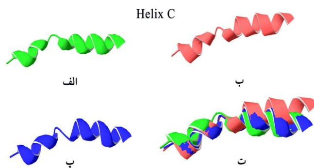
شکل 10 هم‌ردیفی ساختاری مارپیچ C: الف: ساختار مارپیچ C در لحظه اول، ب: ساختار مارپیچ C در لحظه میانی، پ: ساختار مارپیچ C در لحظه پایانی، ت: هم‌ردیفی ساختاری مارپیچ C در لحظات اول، میانی و پایانی
