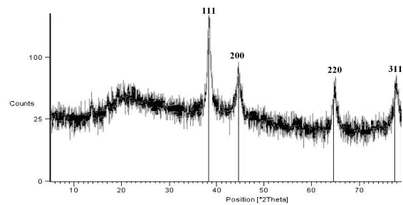
شکل ۲ آنالیز XRD حاصل از نمونه‌های سنتزکننده نانوذرات طلا
