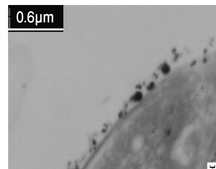
شکل ۳ میکروگراف‌های TEM به‌دست آمده از نانوذرات تولیدشده توسط Streptomyces sp. ERI-3 (الف) نانوذرات سنتز شده به صورت خارج سلولی (ب) نانوذرات سنتز شده به صورت متصل به سطح سلول
