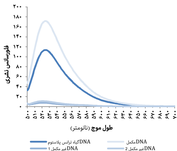
نمودار ۲) شناسایی DNA ترانس پلاستوم توتون با استفاده از نانوحسگر بر پایه گرافن اکسید و کاوشگر ژن گزینشگر aadA
