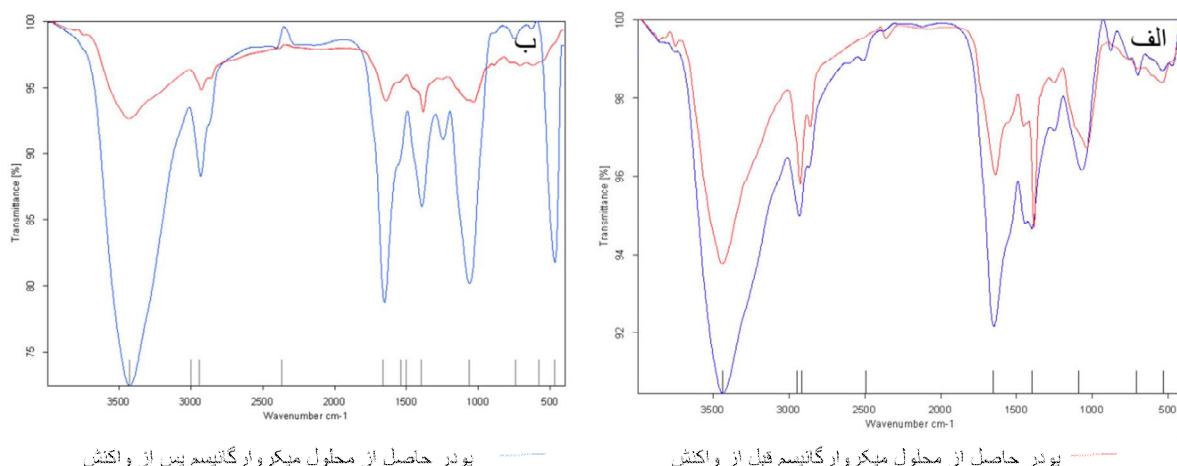
شکل 5. طیف‌های FTIR ثبت‌شده از ساکارومایسس سرویزیه (الف) و کولتوتریکوم گلوَسپوریویدس (ب) قبل و پس از واکنش
