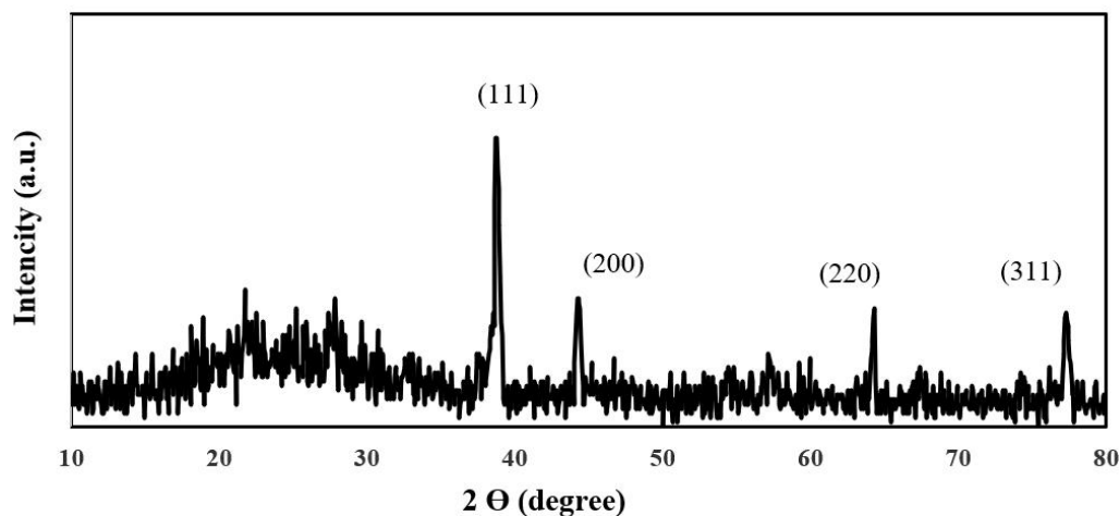
شکل 3 الگوی پراش اشعه ایکس XRD نانوذرات نقره سنتز شده با عصاره بذر گیاه خارخاسک
