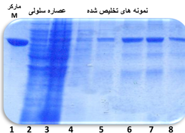
شکل ۳) ژل SDS-PAGE تخلیص پروتئین IP3BD با ستون کروماتوگرافی تمایلی M- مارکر پروتئین (۶۲ کیلو دالتون) - ۲- عصاره سلول قبل القا ۳- عصاره سلول بعد از القا ۴ تا ۸- نمونه‌های تخلیص شده به ترتیب خروج از ستون
