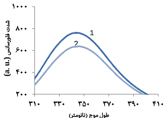
نمودار ۱) طیف نشری فلورسانس ذاتی پروتئین IP3BD در حضور و عدم حضور لیگاند IP3 طیف ۱ در عدم حضور لیگاند IP3 و طیف ۲ در حضور لیگاند IP3 است.
