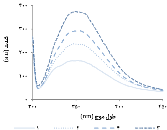
نمودار ۲) طیف فلورسانس ذاتی لوسیفرازهای وحشی و جهش‌یافته‌ها (۱: آنزیم وحشی، ۲: ERR، ۳: ERR/I 232 R، ۴: ERR/Q 35 R/I 182 R/I 232 R) تحت شرایط بافر (pH برابر ۷/۸)، ۵۰ میلی‌مولار تریس، دمای ۲۵°C با غلظت پروتئین ۰/۲ میلی‌گرم بر میلی‌لیتر و طول موج تهییج ۲۹۵ نانومتر
