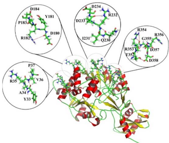
شکل ۲ (a): مدل‌سازی جایگاه‌های جهش. ساختار آنزیم لوسیفراز و جایگاه‌های اسیدآمینه‌های جهش‌داده‌شده با استفاده از Swiss Model Server
