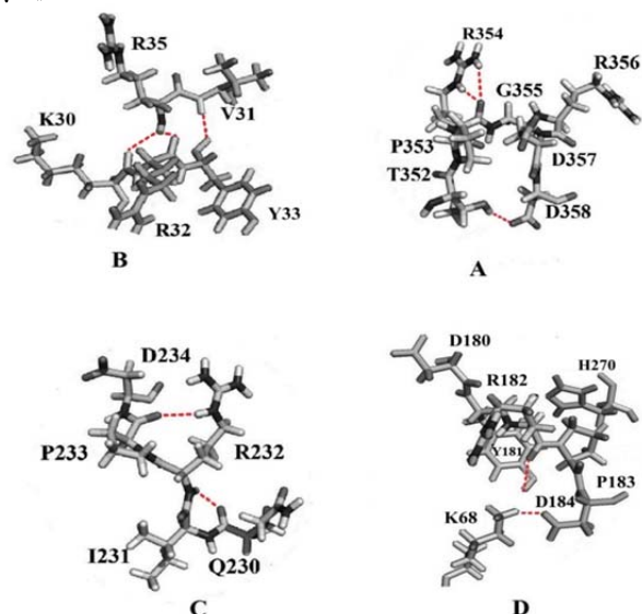
شکل ۳) انواع جهش‌های ایجادشده در محل‌های: (A) ERR, (B) Q 35 R, (C) I 232 R, (D) I 182 R و پیوندهای ایجادشده با اسیدآمینه‌های مجاورشان که با استفاده از PIC-Server به دست آمده است
