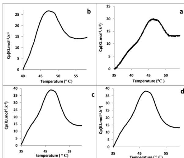
نمودار ۳ (a): ترموگرام‌های به‌دست‌آمده از مطالعه کالریمتری روبشی تفاضلی پروتئین وحشی و جهش‌یافته‌ها: a: آنزیم وحشی، b: ERR، c: ERR/I 232 R، d: ERR/Q 35 R/I 182 R/I 232 R (میزان ظرفیت گرمایی این پروتئین‌ها در جهت محور Y جابه‌جا شده است تا بدین ترتیب این ترموگرام‌ها بهتر نشان داده شوند)
