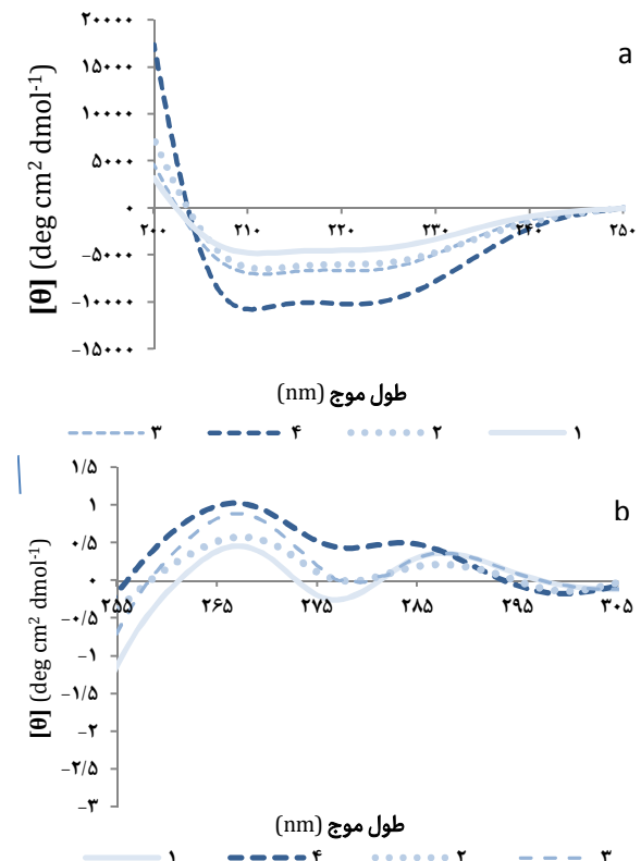
نمودار ۱) (a): طیف‌های دورنگ‌نمایی دورانی در ناحیه دور فرابنفش برای بررسی ساختار دوم پروتئین‌های وحشی و جهش‌یافته (۱: آنزیم وحشی، ۲: ERR، ۳: ERR/I 232 R، ۴: ERR/Q 35 R/I 182 R/I 232 R)، (b): طیف‌های دورنگ‌نمایی دورانی در ناحیه نزدیک فرابنفش برای بررسی تغییرات موضعی ساختار سوم پروتئین‌های وحشی و جهش‌یافته (۱: آنزیم وحشی، ۲: ERR، ۳: ERR/I 232 R، ۴: ERR/Q 35 R/I 182 R/I 232 R)
