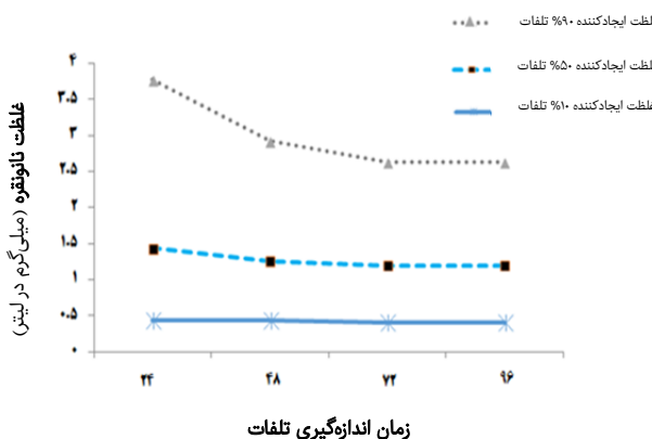
نمودار ۶) روند ایجاد تلفات در ماهی گورخری با افزایش غلظت نانوذرات نقره شیمیایی طی افزایش زمان مجاورت
