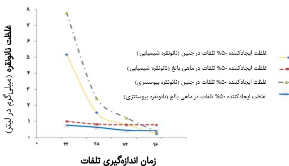
نمودار ۵) مقایسه غلظت ایجادکننده LC_{50} در جنین و بالغ ماهی گورخری طی افزایش زمان مجاورت با نانوذرات نقره شیمیایی (AgNPs) و زیست‌تولیدشده توسط جلبک دریایی قهوه‌ای
