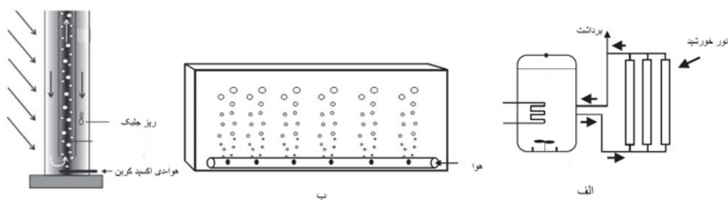
شکل ۴ (الف) انواع زیست‌واکنش‌گاه‌های نوری بسته: لوله‌ای (الف)، صفحه تخت (ب) هوای بالارونده (ج) [22]
