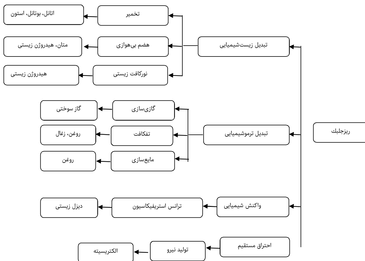
شکل ۱) فرآیندهای تولید انرژی از ریزجلبک [13]
