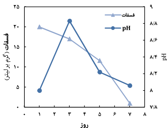
نمودار (۲) منحنی کاهش غلظت نیترات و pH برحسب روز توسط کلرلا سالینا
