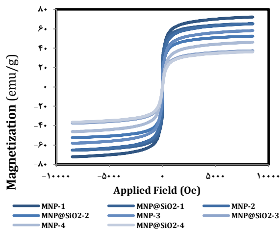
نمودار ۱) لوپ‌های هیستریزس نانوذرات مغناطیسی ساخته شده با پروتکل‌های مختلف
