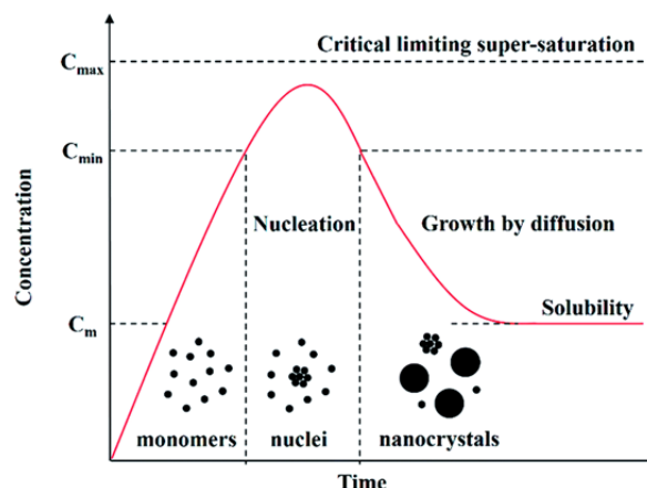
نمودار ۵) نمودار هسته‌زایی و رشد هسته نانوبلورها (نمودار LaMer)
