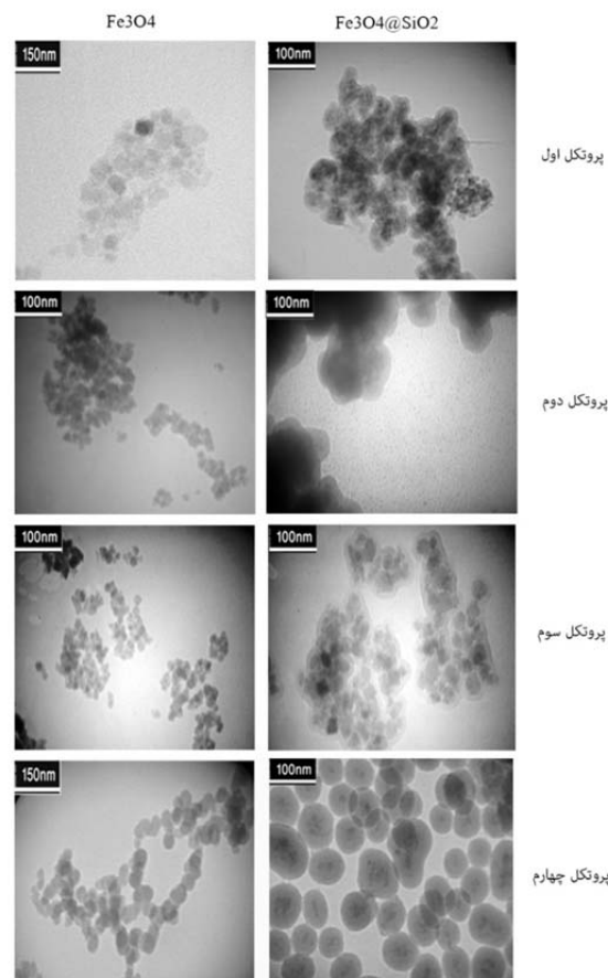
شکل ۱) تصاویر میکروسکوپ الکترونی نانوذرات سنتز شده با پروتکل‌های مختلف (ستون سمت چپ: Fe_3O_4 ، ستون سمت راست: Fe_3O_4@SiO_2 ) الف) نانوذرات سنتز شده با استفاده از پروتکل اول ب) نانوذرات سنتز شده با استفاده از پروتکل دوم ج) نانوذرات سنتز شده با استفاده از پروتکل سوم د) نانوذرات سنتز شده با استفاده از پروتکل چهارم ضخامت لایه سیلیکا و نیز میزان توده‌ای شدن نانوذرات و پراکندگی آنها در شکل قابل مشاهده است.
