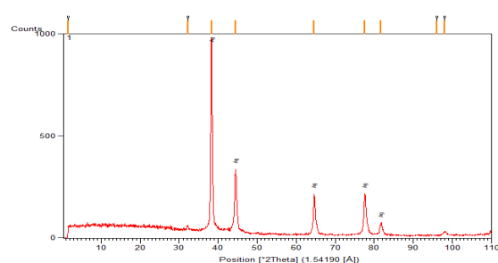
نمودار ۲) طیف XRD نانوذرات نقره بلوط
