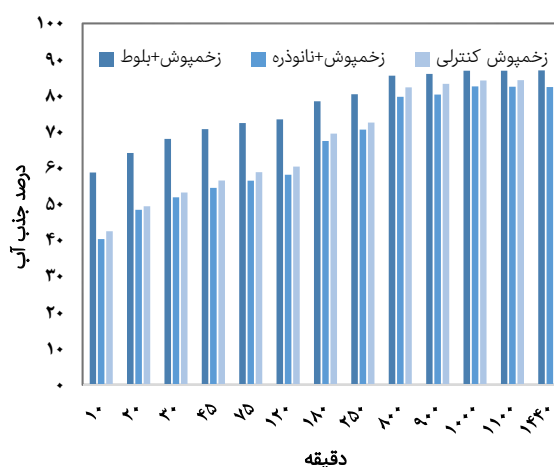
نمودار ۵) درصد جذب آب برای سه نمونه به مدت ۲۴ ساعت. از زخم‌پوش بدون نانوذره و عصاره به‌عنوان نمونه کنترل استفاده شد.
