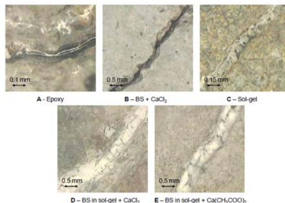
شکل ۴) A: یک ترک ترمیم‌شده با اپوکسی را نشان می‌دهد که با اپوکسی کاملاً پر شده است، B: یک ترک با BS + CaCl_2 ترمیم‌شده را نشان می‌دهد، در این حالت چون باکتری در برابر قلیای بالای بتن محافظت نشده‌اند، رسوبات کلسیم کریستال باکتریایی تولید نشده است. در شکل D-۴ و E-۴ باکتری همراه با سیلیکاژل استفاده شده و ترک‌ها ترمیم و پر شده‌اند. در شکل C-۴ حالتی که فقط سولژل استفاده شود در حین خشک‌شدن ترک‌هایی ایجاد می‌شود که حفاظت کامل نمی‌تواند ایجاد کند. در شکل D-۴ و E-۴ که سول ژل و کلسیم کریستال یا کلسیم استات استفاده شود و در محلول اوره- کلسیم بعد از پرکردن ترک‌ها توسط ژل و باکتری غوطه‌ور شود، در این حالت رسوب کلسیم کریستال به وسیله باکتری ایجاد شده و ترک‌ها کاملاً پر می‌شوند.
