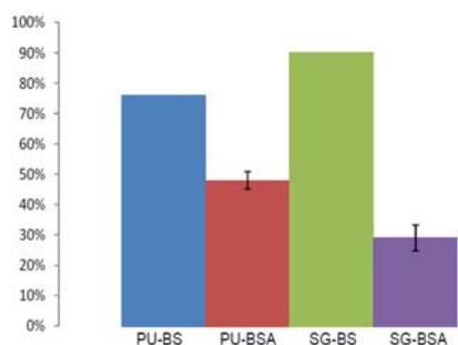
نمودار ۱) تغییرات استحکام ناشی از فرآیند خودترمیمی بتن با پلی‌یورتان سیلیکا ژل، باسیلوس اسفریکوس و باسیلوس اسفریکوس مرده (اتوکلاوی)
