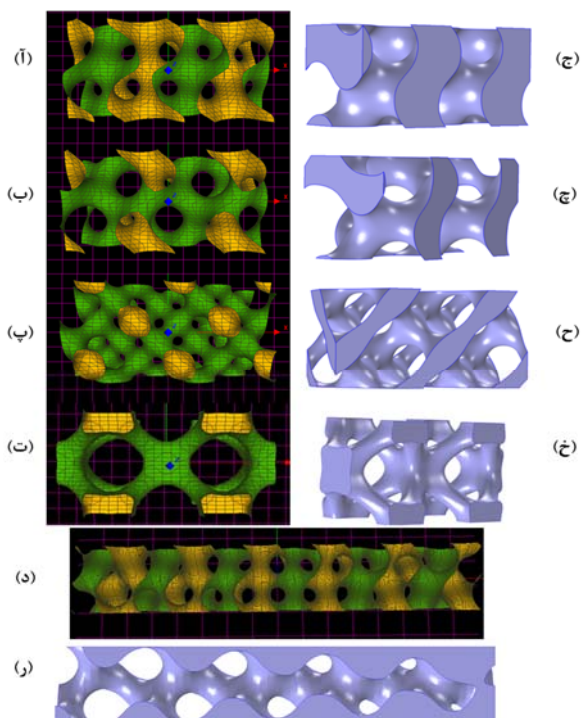
شکل ۱) رویه‌ها و داربست‌های طراحی‌شده (آ و ج: جیروید)، (ب و د: جیروید پر تخلخل)، (پ و ح: دیاموند)، (ت و خ: IWP) و (د و ر): با شیب تخلخل
