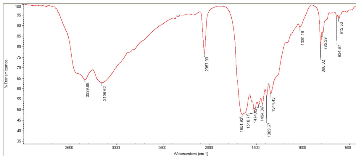
شکل 1- طيف FTIR کربن نیتريد گرافيتي سنتز شده.
