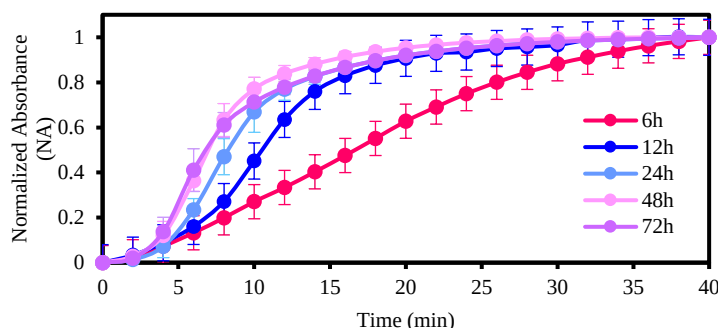
شکل ۲ منحنی کدورت سنجی هیدروژل آمینوئیل انحلال یافته در زمان های مختلف.
