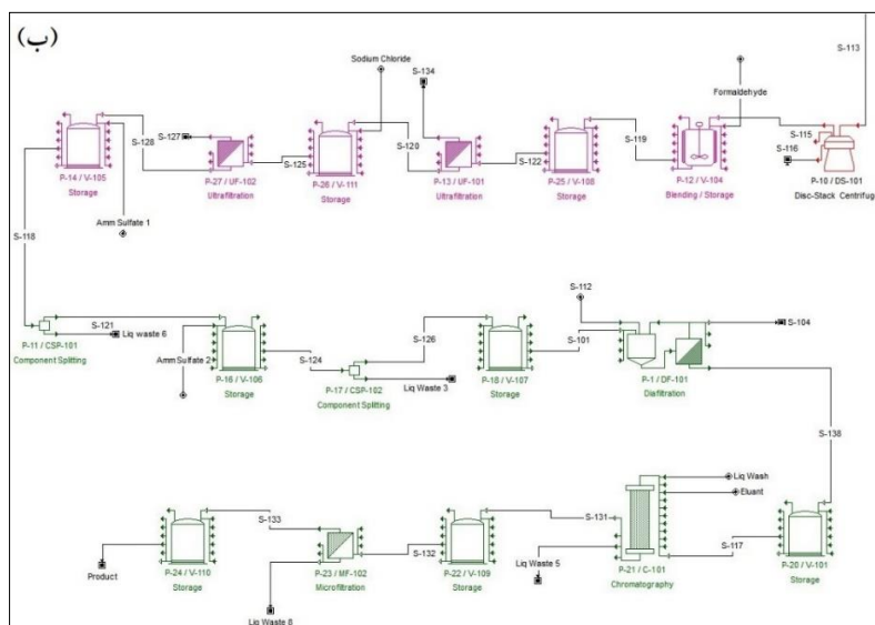
شکل ۱ نمودار جریان فرآیند بالادستی (الف) جریان فرآیند پایین‌دستی (ب) تولید توکسویید دیفتتری (فرآیند واقعی).
