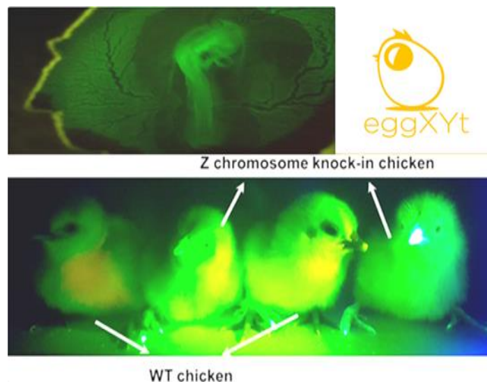
شکل ۳ تصویری شماتیک از تعیین جنسیت تخم مرغ با فناوری کریسپر. جنین ۲,۵ روزه نر که تحت تابش نور فلئورسنت به رنگ سبز می درخشد (بالا- چپ)، لوگوی شرکت مربوطه (بالا- راست)، تفکیک جوجه های نر ترانس ژنیک از جوجه های ماده طبیعی که با درخشش تحت تابش نور فلئورسنت، قابل تشخیص است (پایین).
