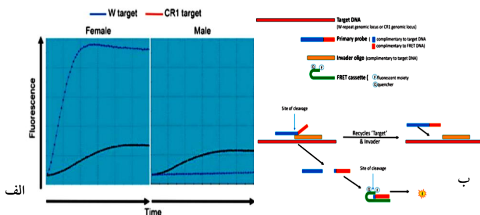
شکل ۴ راست- تصویری از مکانیسم تشخیص جنسیت جنین‌های جوجه. (الف) اجزای نوکلئیک اسیدی مورد نیاز در سنجش جنسیت، (ب) ایجاد سیگنال فلورسانس. چپ- نمودارهای فلورسانس نشر شده برای توالی تکراری W (توالی ویژه کروموزوم جنسی ماده) به رنگ آبی و توالی تکراری CR1 (توالی مشترک کروموزوم جنسی نر و ماده) به رنگ قرمز [۲۷].
