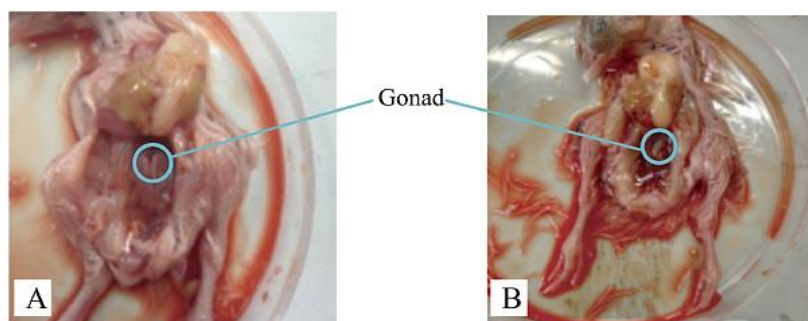
شکل ۸ مورفولوژی گنادهای جنسی جنین‌های جوجه. جوجه نر در تصویر A و جوجه ماده در تصویر B قابل به مشاهده است [۳۷].
