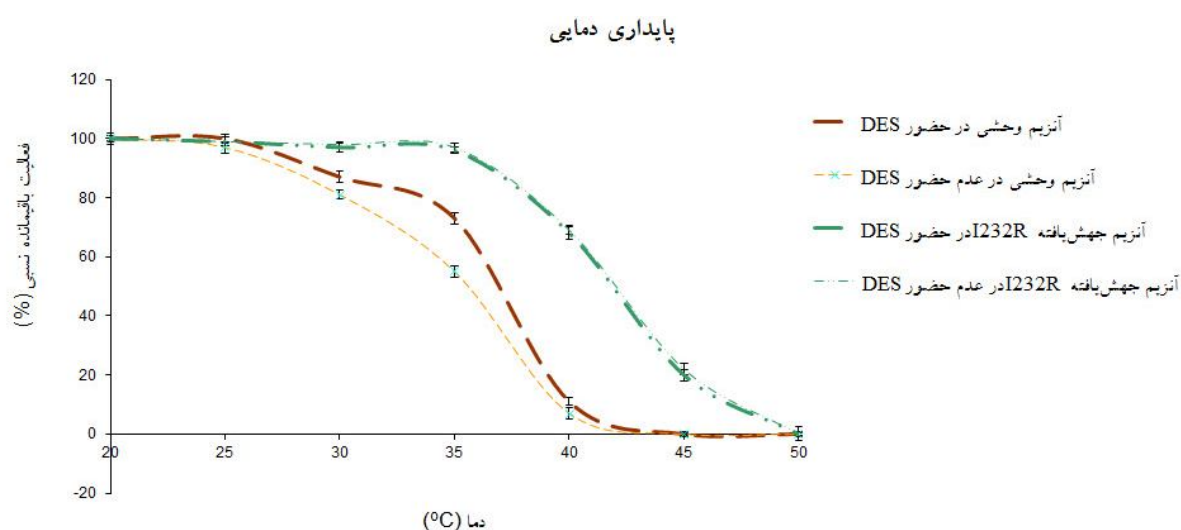
شکل 4 پایداری دمایی آنزیم‌های وحشی و جهش یافته \text{I}^{232}\text{R} - \text{E}^{354}\text{R}/\text{Arg}^{356} در حضور و عدم حضور حلال DES. آنزیم جهش یافته \text{I}^{232}\text{R} - \text{E}^{354}\text{R}/\text{Arg}^{356} در شکل به اختصار \text{I}^{232}\text{R} نوشته شده است.
