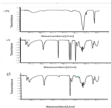
شکل 3 نتایج FTIR از الف- پوست میگوی خام، ب- پوست میگوی تخمیر شده با باسیلوس آلتی شودنیس پس از سه روز در دمای 37 درجه سلسیوس، ج- پوست میگوی تخمیر شده با سویه باسیلوس لیکنی فورمیس پس از سه روز در دمای 37 درجه سلسیوس.
