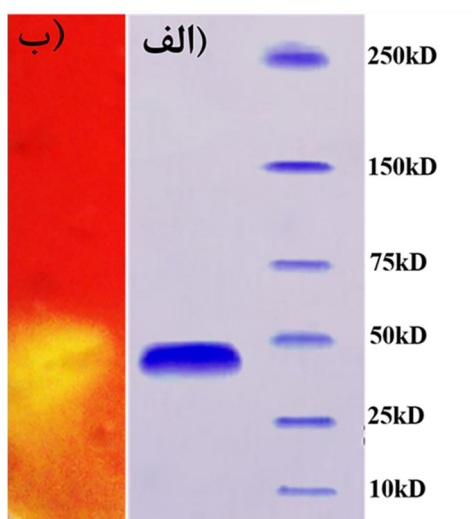
شکل 7 الف الکتروفورز ژل پلی آکریل سدیدم دودسیل سولفات (SDS-PAGE) نمونه مایع روی کشت باسیلوس آلتی‌شودنیس روی کشت جامد پوست میگو پس از تیمار حرارتی و تغلیظ آن با سولفات آمونیوم؛ ب- آنالیز زیموگرام نمونه روی ژل حاوی کیتین کلوتیدال رنگ‌آمیزی‌شده با کنگورد.
