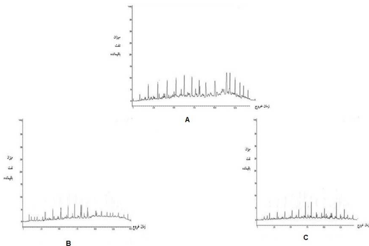
شکل 3 طیف‌های گاز کروماتوگرافی تجزیه نفت خام توسط دو سویه برتر (A): شاهد نفت بدون باکتری (B): سویه 3-1-4-1 BA و (C) سویه 1-4-1-4 BA
