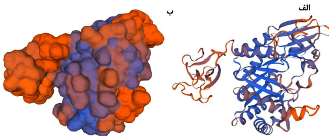
شکل 4- ساختار سه بعدی پیش بینی شده کیتیناز از F. merquensis الف-مدل کارتونی و ب- مدل سطحی
