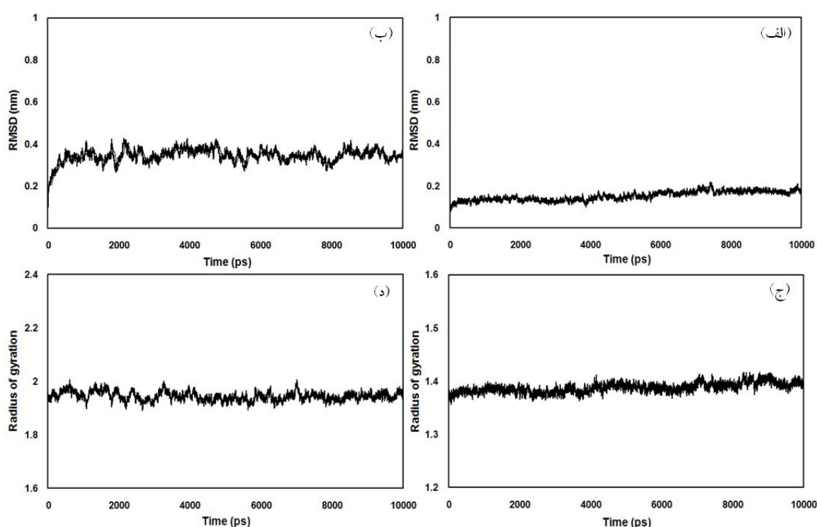
شکل 8 بررسی پایداری ساختار شبیه‌سازی شده. تغییرات RMSD (الف) و VEVhh1 (ب) VEGF طی 10 نانوثانیه شبیه‌سازی.
