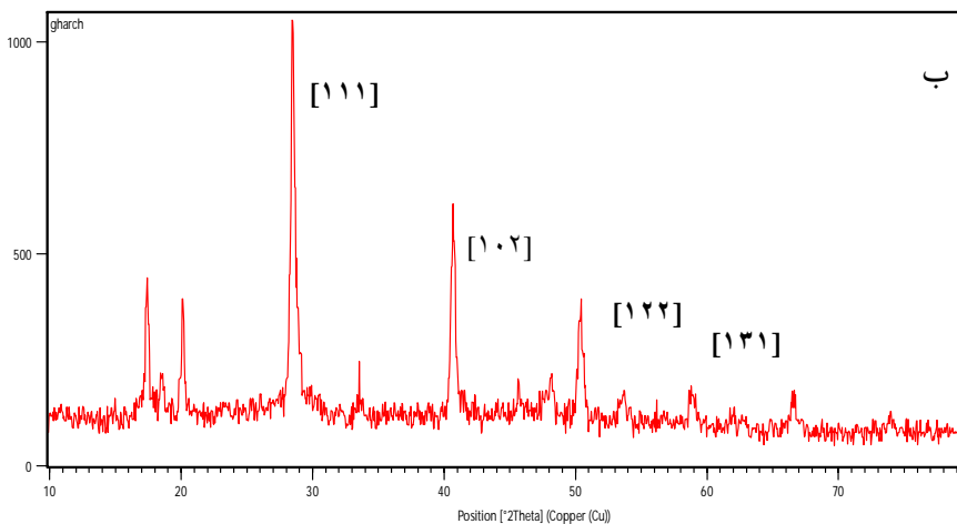
شکل 3. نمودار الگوی XRD به دست آمده از نانوذرات بیوسنتز شده توسط ساکارومایسس سرویزیه (الف) و کولتوتریکوم گلوسپوریویدس (ب)
