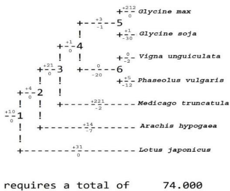
شکل ۲. روند ایجاد و از بین رفتن خانواده‌های miRNA در درخت روابط فیلوژنتیکی گونه‌های مورد مطالعه به شیوه مدل پیشینه پارسیمونی دولو. اعداد نمایش داده شده بر روی مسیرهای تکاملی نشان دهنده تعداد خانواده‌های ایجاد شده (+) و از بین رفته (-) در طول مسیر تکاملی را نمایش می‌دهد.
