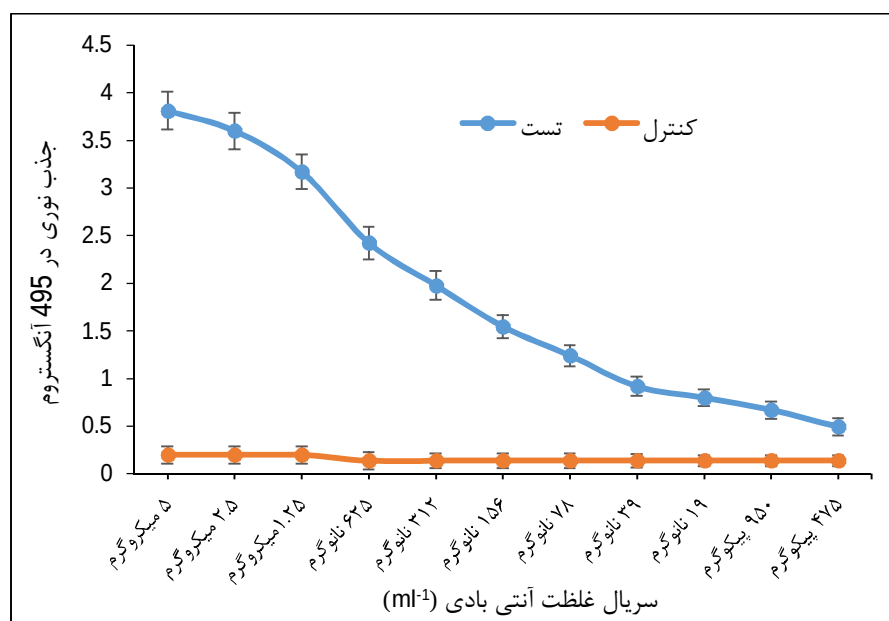
نمودار 1 نمودار الایزا غیرمستقیم آنتی بادی موشی با آنتی ژن نو ترکیب BoNT/B-HcC، نمونه کنترل شامل آنتی ژن BoNT/A و نمونه آزمون شامل آنتی ژن BoNT/B، نتایج نشان داد که آنتی بادی موشی تا غلظت 475 پیکوگرم از آنتی ژن BoNT/B را در مقایسه با کنترل شناسایی کند.
