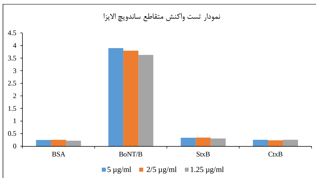
نمودار 5 بررسی میزان اختصاصیت سازه ساندویچ الایزا در شناسایی BoNT/B، نتایج مقایسه آماری واکنش متقاطع ساندویچ الایزا در شناسایی سم BoNT/B در مقایسه با دیگر سموم نشان داد که نتایج OD در سموم متفرقه با نمونه‌های شاهد نزدیک بوده است و با سم BoNT/B از لحاظ آماری تفاوت معناداری دارند.
