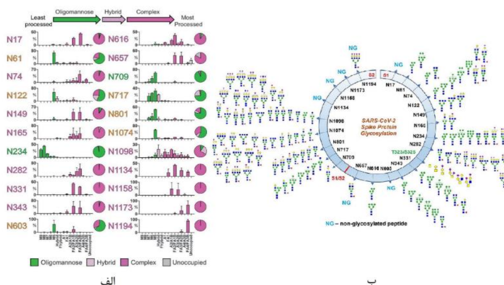
شکل ۵ دو پروفایل قندی مختلف از پروتئین اسپایک کروناویروس جدید (اقتباس شده از [۱۸, ۱۹]).
