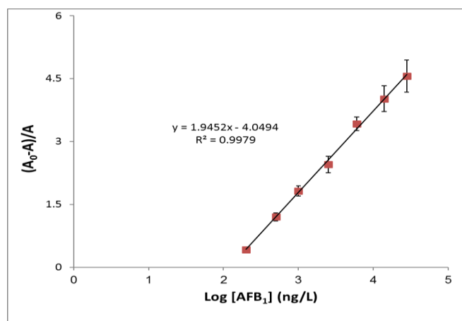
شکل ۶ بررسی عملکرد آبتاسنسور در نمونه سرم. حرف A عدد اگریگاسیون بعد از اضافه کردن AFB 1 و A 0 عدد اگریگاسیون قبل از اضافه کردن AFB 1 می باشد.
