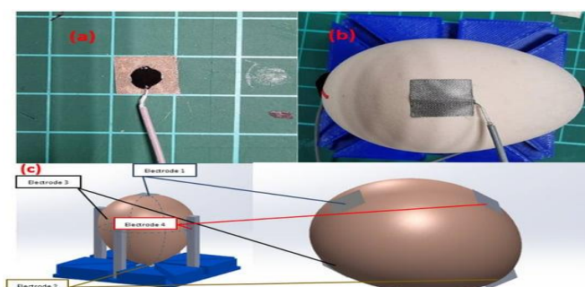
شکل ۱۰ (a) مراحل تعیین جنسیت جنین جوجه به روش طیف سنجی امپدانس. (b) اپوکسی کربن بر روی چسب پارچه‌ای رسانا به ابعاد ۱۰×۱۰ میلی‌متر مربع ریخته می‌شود. (c) بر روی نقاط مشخص شده روی تخم‌مرغ با استفاده از کابل کوکسیال RG-13 ۱ میلی‌متری در موقعیت‌های تعیین شده برای الکترودها چسبانده می‌شود [۴۴].
