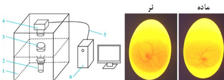
شکل ۷ راست- تصاویر گرفته شده توسط دوربین که نشانگر جنین‌های نر و ماده است. چپ- تصویری از سامانه تصویربرداری ماشینی. ۱، اتاق تاریک؛ ۲، منبع نور؛ ۳، تخم‌مرغ؛ ۴، دوربین صنعتی؛ ۵، کابل داده و ۶، سیستم پردازشگر [۳۷].
